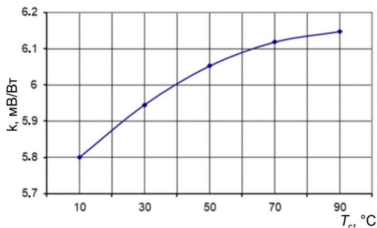
Рис. 6. Температурна залежність вольт-ватної чутливості тепломіра розмірами 40 × 40 мм
